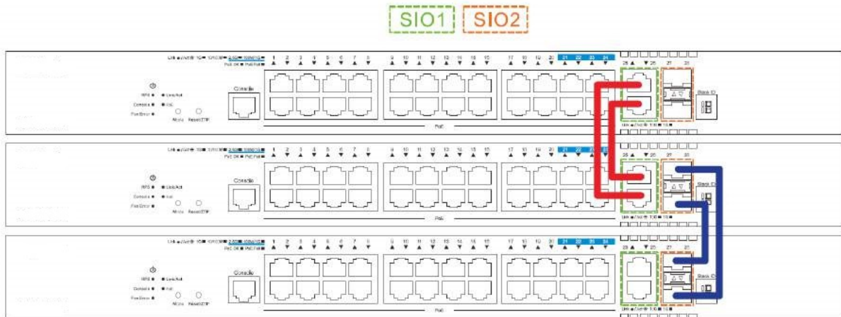
Рис. 5 – Линейная топология (нечетное количество коммутаторов, с использованием 4 портов).
