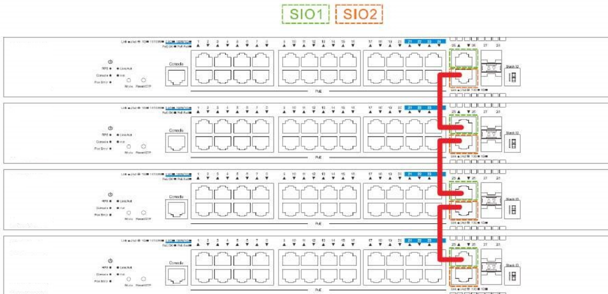
Рис. 1 – Линейная топология (четное количество коммутаторов, с использованием 2 портов).
